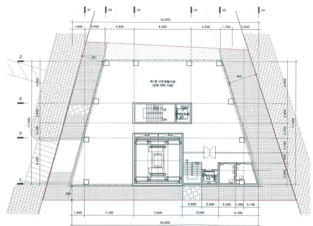
설계도면
